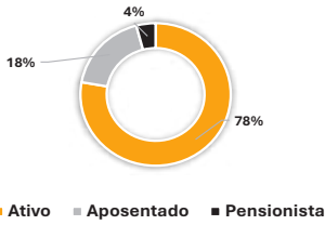
Quadro 10 - Folha Mensal dos Segurados - Remuneração Média
