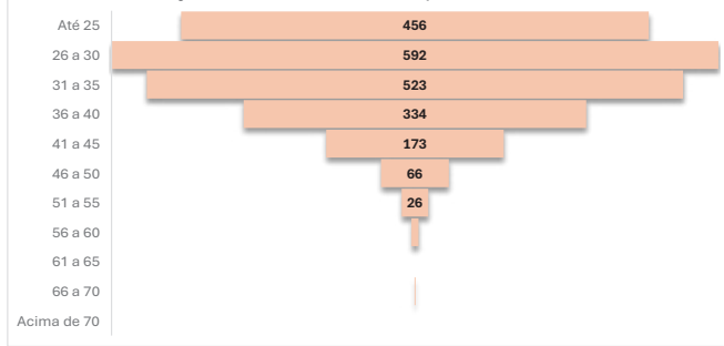
Distribuição dos Servidores Ativos por idade de admissão
