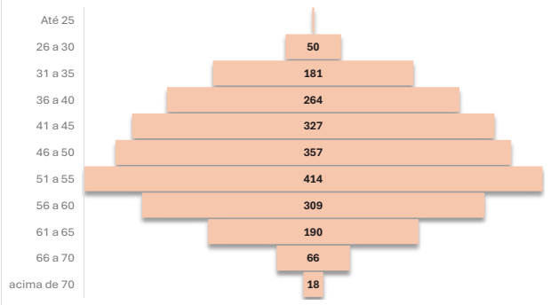
Distribuição dos servidores ativos por faixa etária
